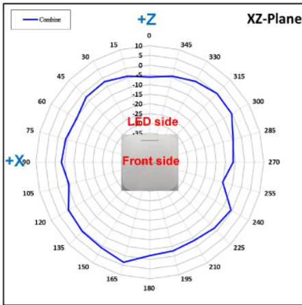
5 GHz Antenna
