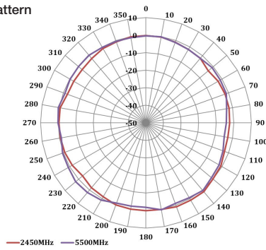
H-Plane Pattern
